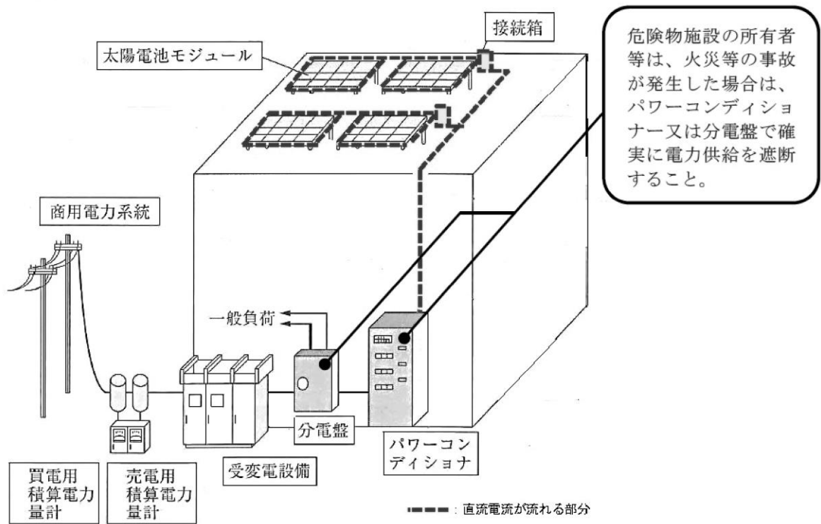
別図 感電防止のための表示が必要な範囲
