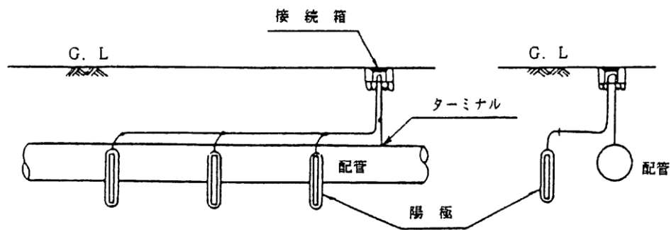
第1-6-3図 流電陽極方式の施工例
