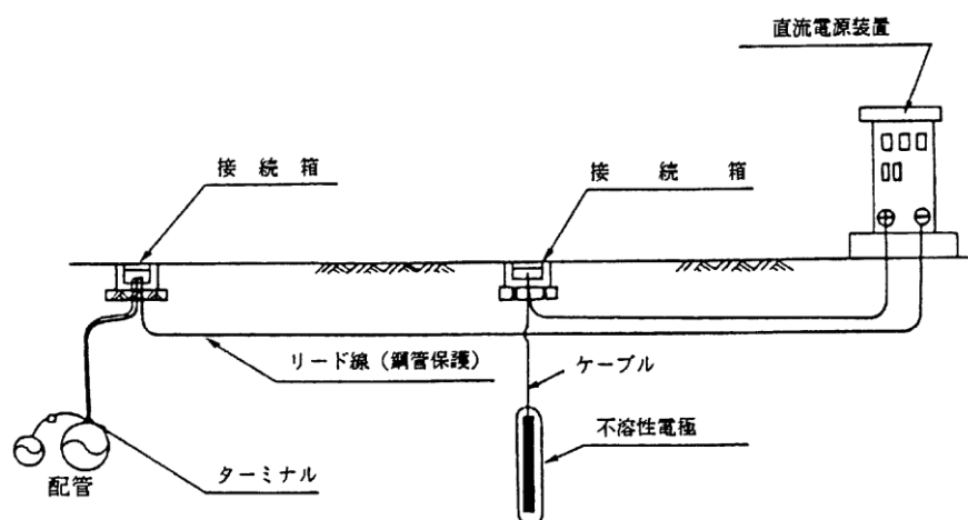
第1-6-4図 外部電源方式の施工例
