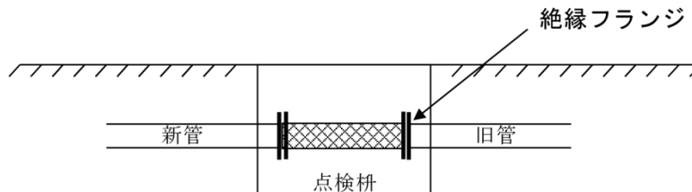
第 1 - 6 - 1 図 絶縁処理が必要な場合の例
