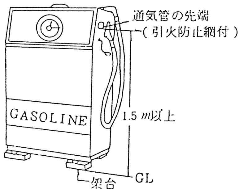
第10-1図 通気管の高さ
