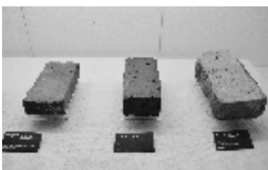
左が中国、中央が韓国、右がドイツで生産された大きさが異なるれんが
